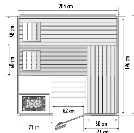
Blockbohle-A Gerade
